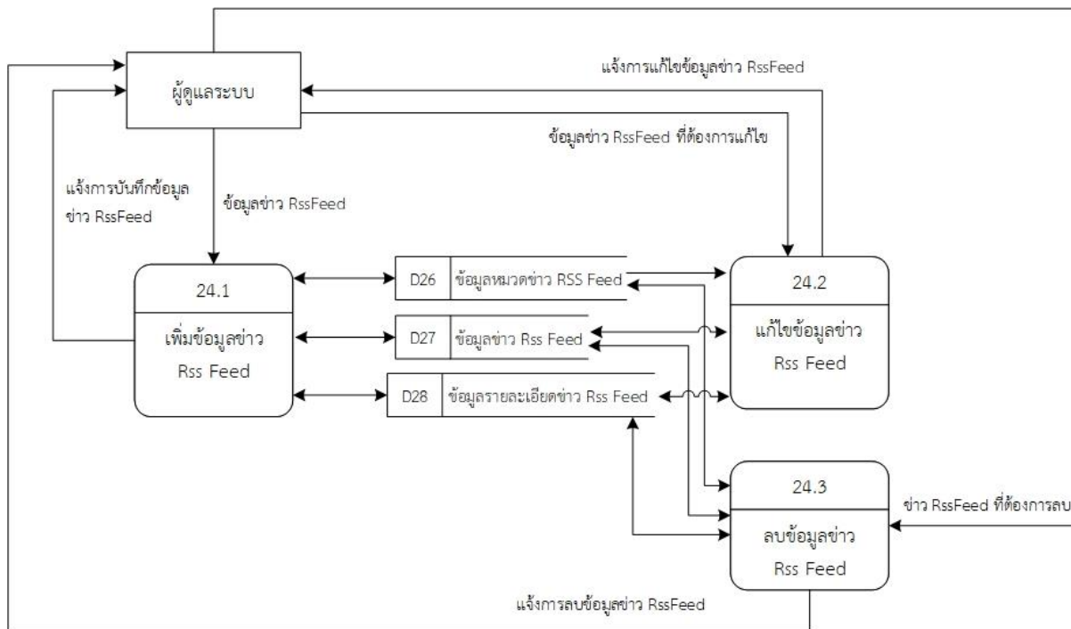
ภาพที่ 75 DFD Process 24 ข่าวสาร RssFeed
