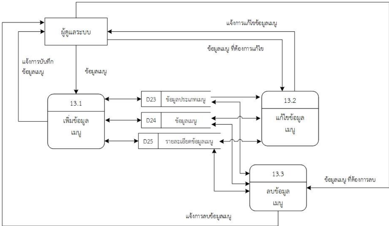
ภาพที่ 64 DFD Process 13 จัดการเมนู
