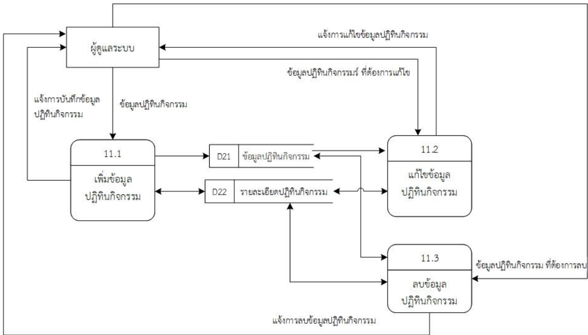
ภาพที่ 62 DFD Process 11 จัดการปฏิทิน
