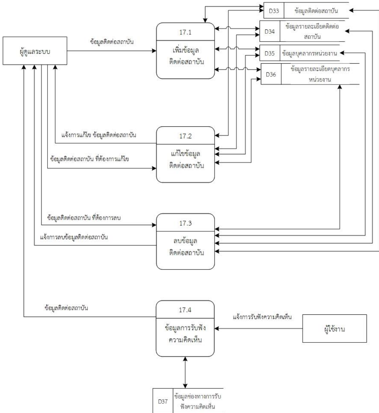
ภาพที่ 68 DFD Process 17 ติดต่อสถาบัน
