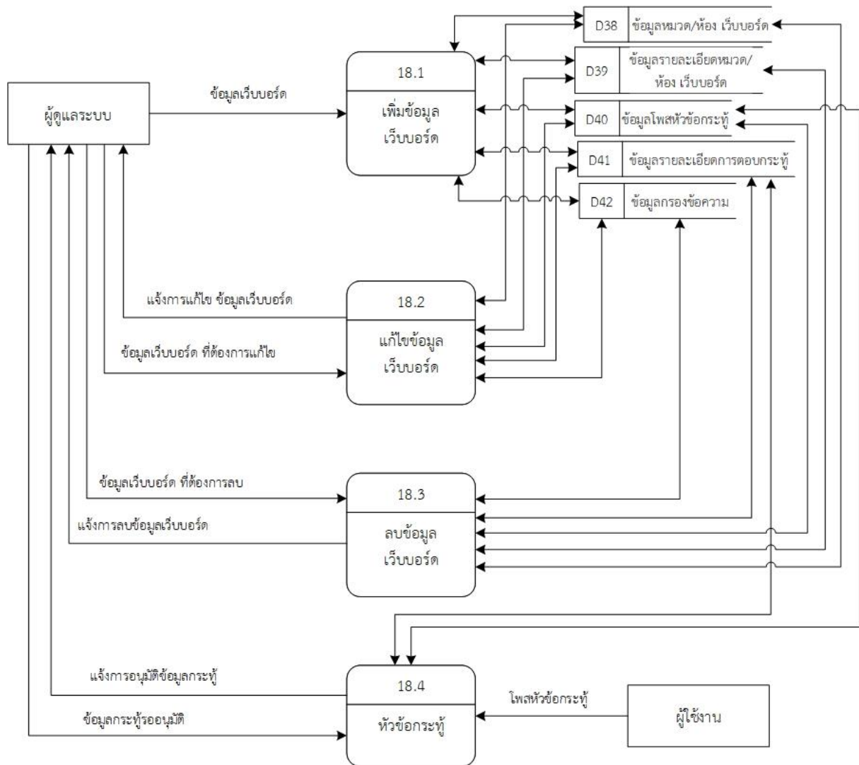
ภาพที่ 69 DFD Process 18 เว็บไซต์
